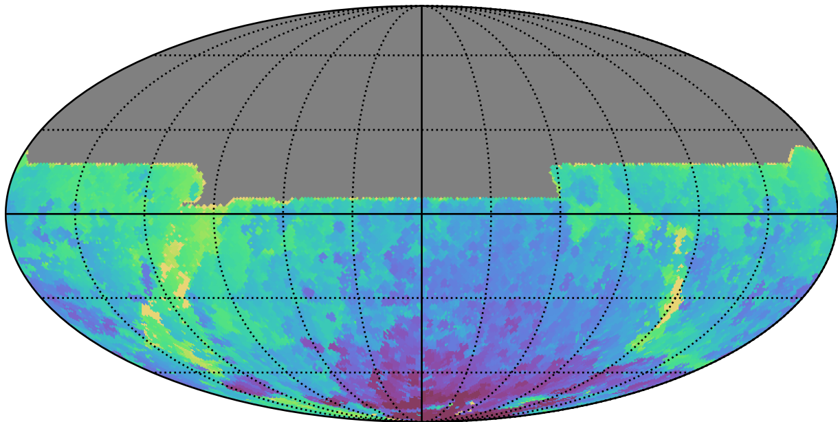
ddf_acor_sf10_lsf15_lsr10_v3.4_10yrs All sky y band: Min HA
