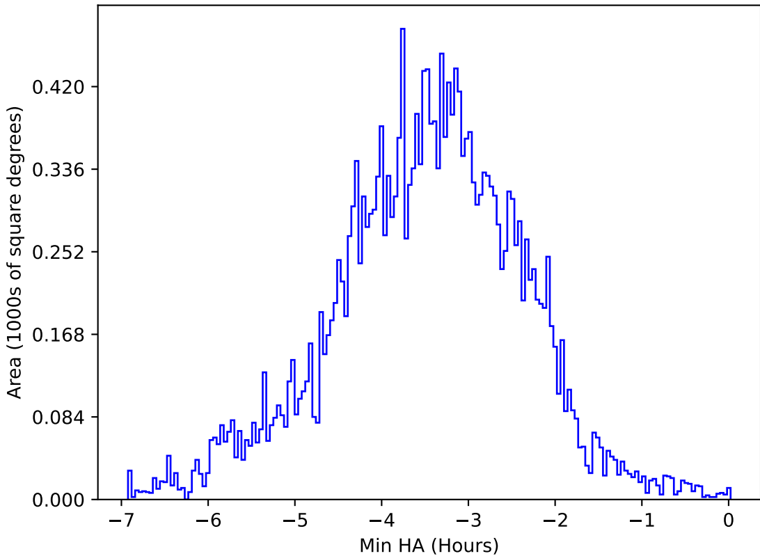
ddf_acor_sf10_lsf15_lsr10_v3.4_10yrs All sky y band: Min HA
