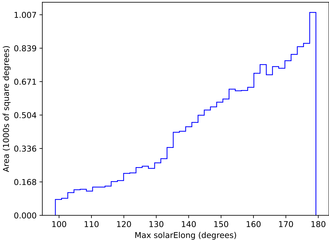
ddf_acor_sf10_lsf15_lsr10_v3.4_10yrs WFD y band: Max solarElong
