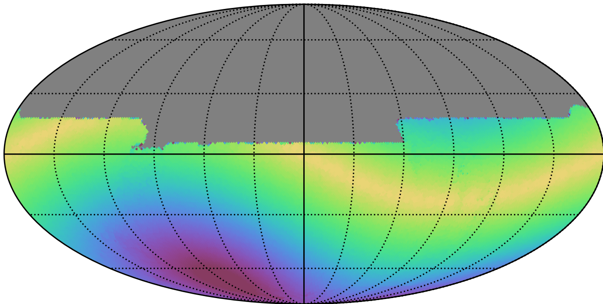
ddf_acor_sf10_lsf15_lsr10_v3.4_10yrs All sky y band: Max solarElong
