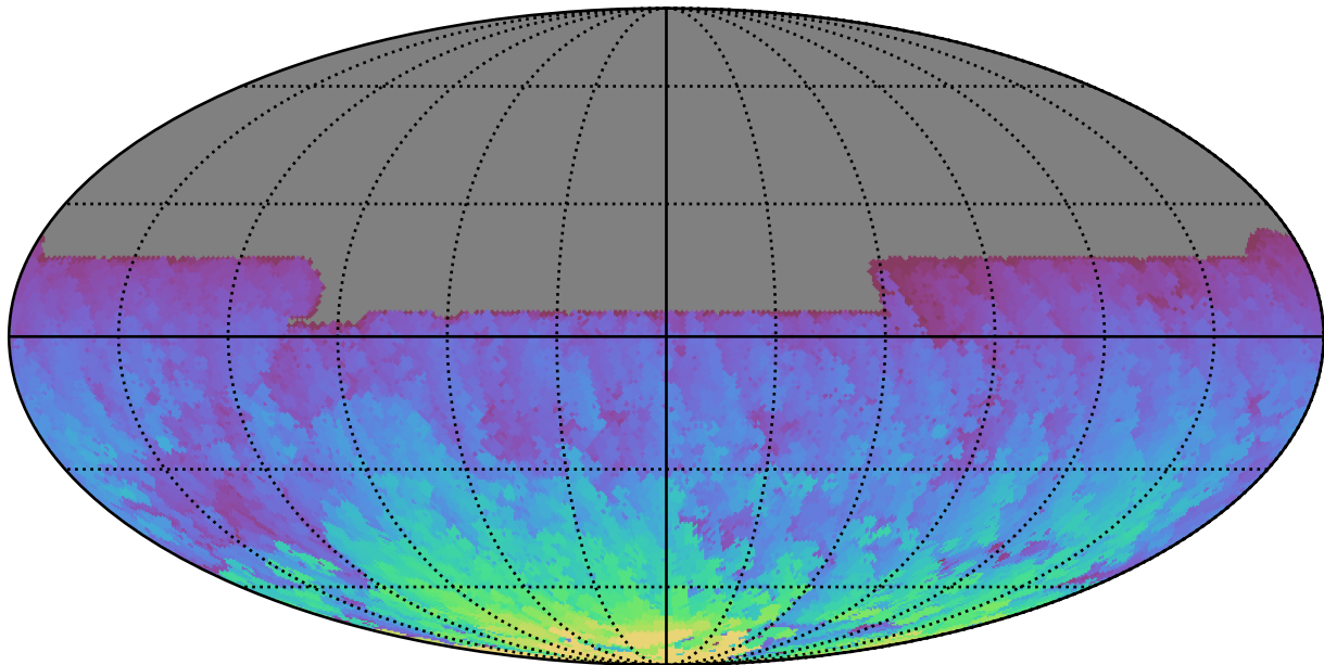
ddf_acor_sf10_lsf15_lsr10_v3.4_10yrs All sky y band: Max HA
