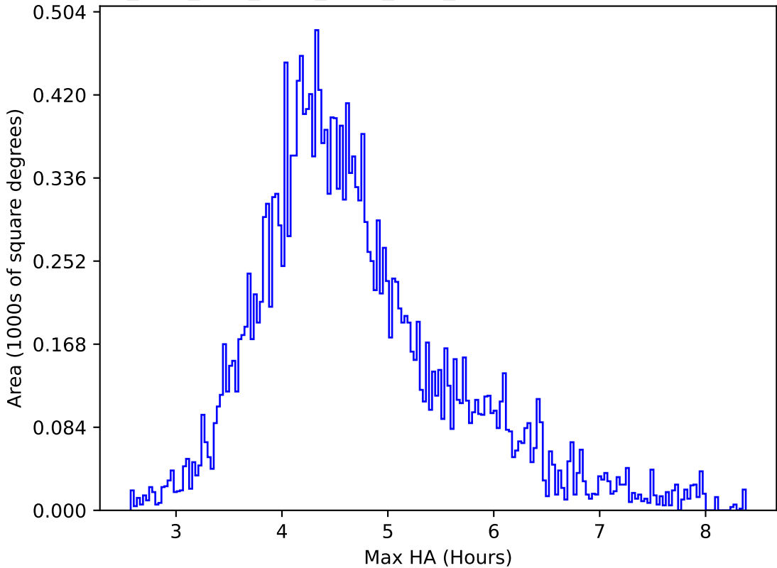
ddf_acor_sf10_lsf15_lsr10_v3.4_10yrs All sky y band: Max HA
