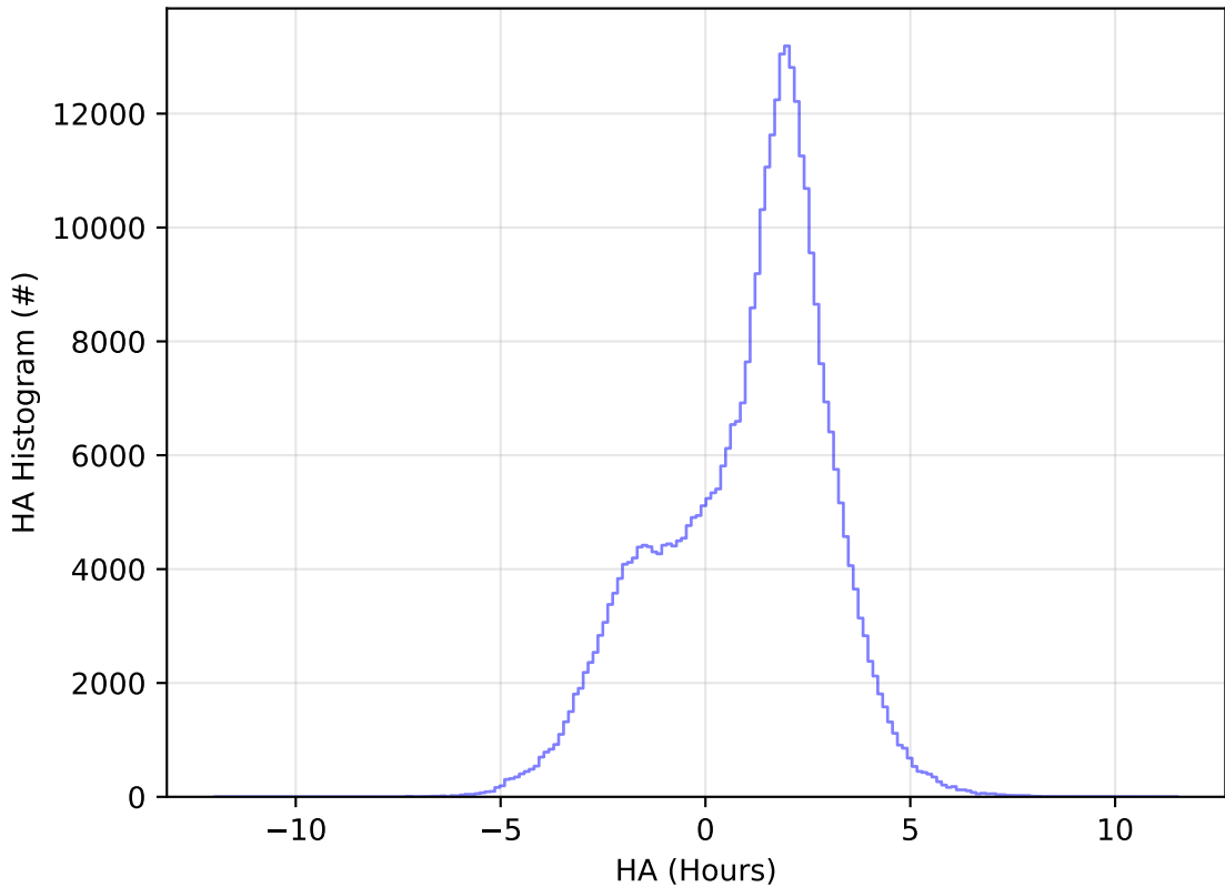
ddf_acor_sf10_lsf15_lsr10_v3.4_10yrs All sky y band: HA Histogram
