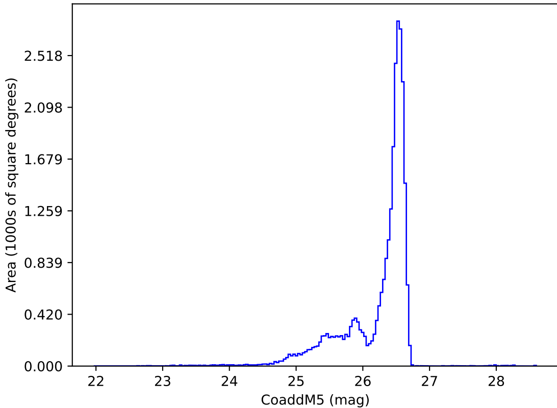
ddf_acor_sf10_lsf15_lsr10_v3.4_10yrs i: CoaddM5
