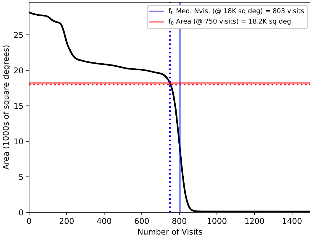
baseline_v3.5_10yrs All sky: f0
