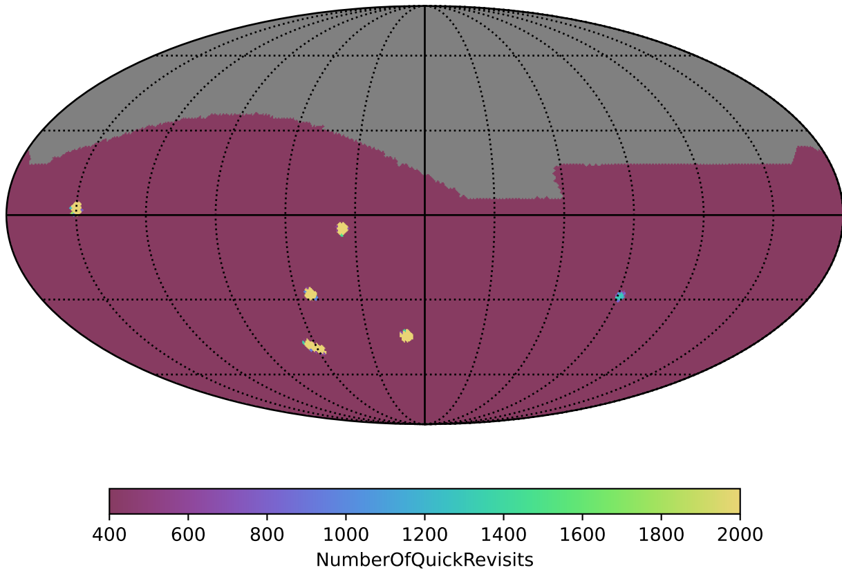
baseline_v3.5_10yrs All sky: NumberOfQuickRevisits
