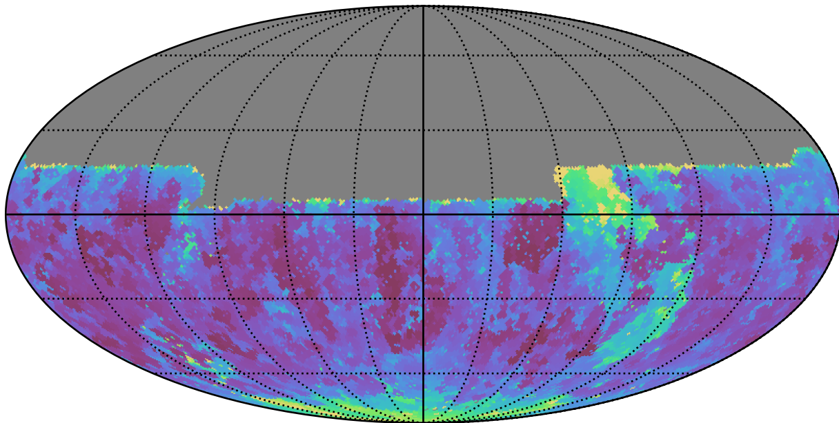
baseline_v3.5_10yrs Yr 1 y band: Min seeingGeom
