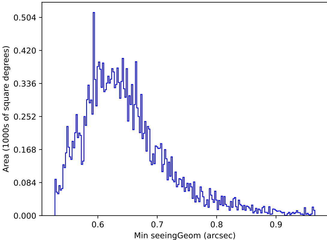
baseline_v3.5_10yrs Yr 1 y band: Min seeingGeom
