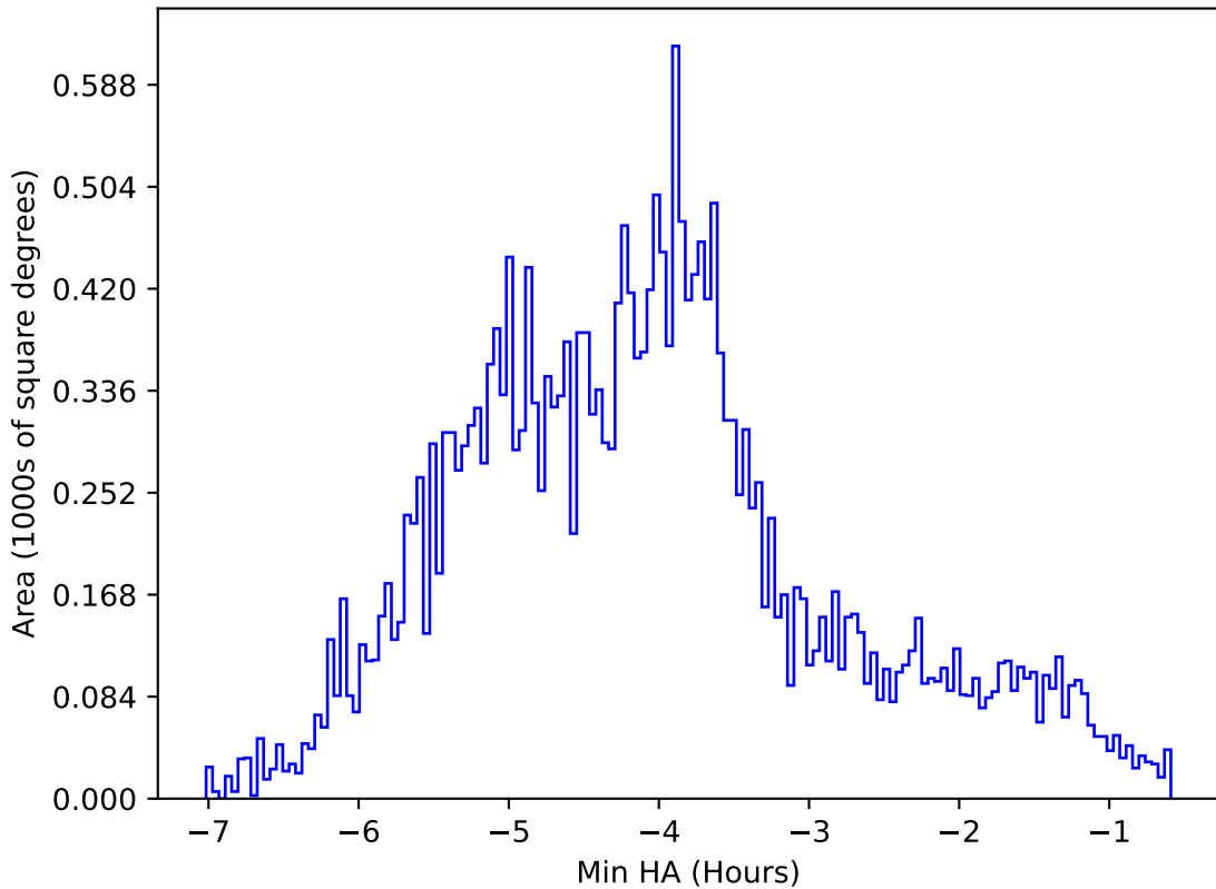
baseline_v3.5_10yrs All sky z band: Min HA
