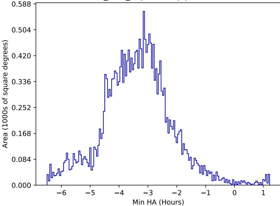
baseline_v3.5_10yrs All sky y band: Min HA
