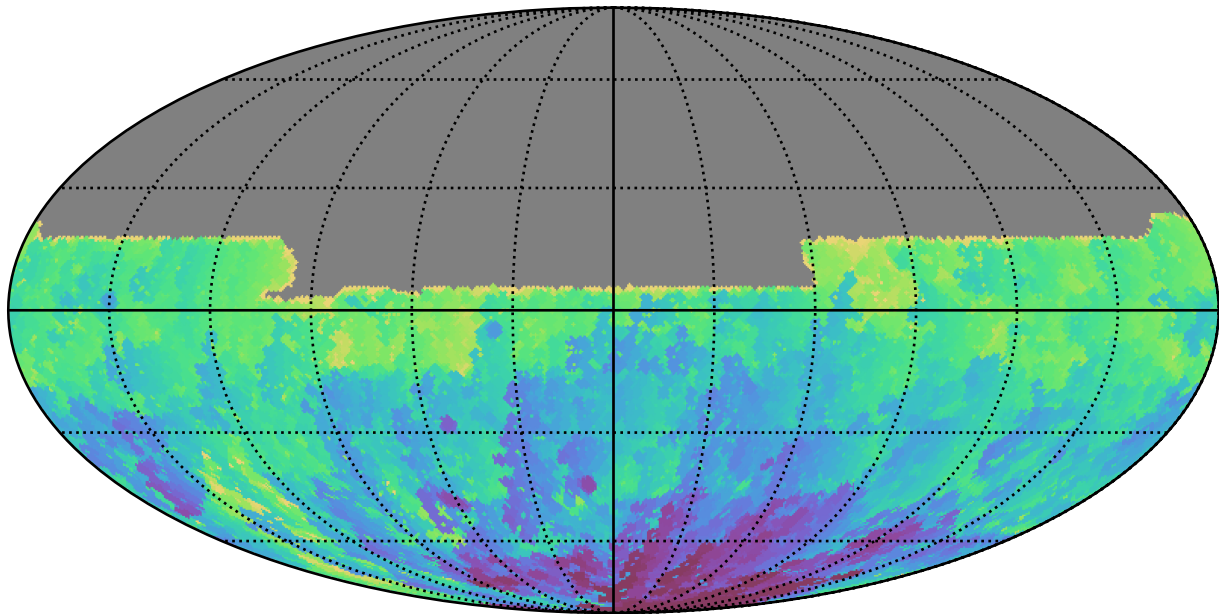
baseline_v3.5_10yrs All sky u band: Min HA
