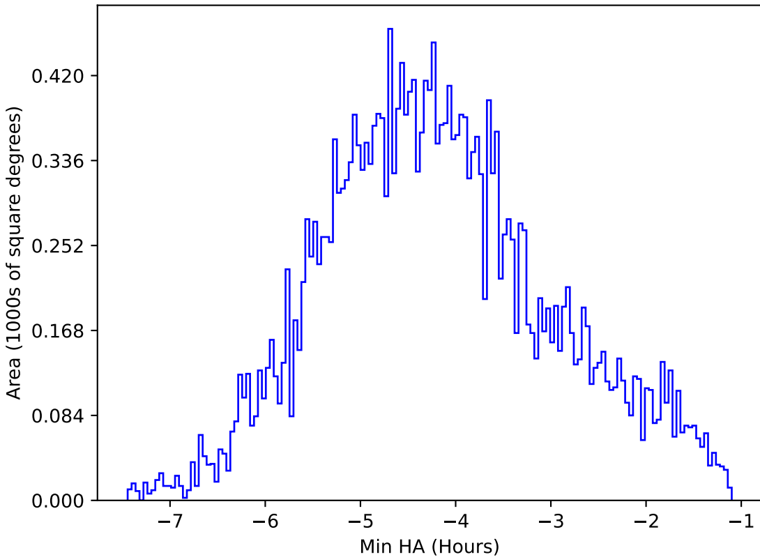
baseline_v3.5_10yrs All sky i band: Min HA
