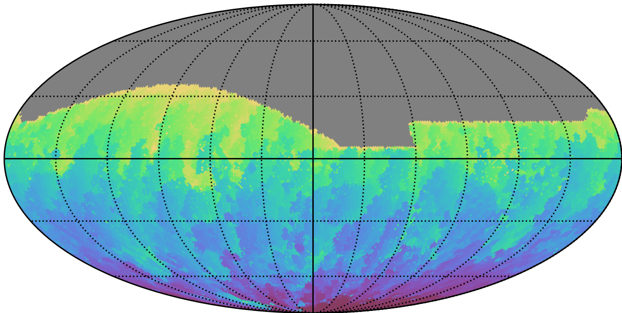
baseline_v3.5_10yrs All sky g band: Min HA
