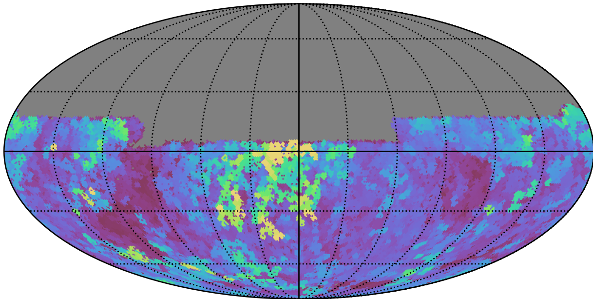
baseline_v3.5_10yrs Yr 1 y band: Max seeingGeom
