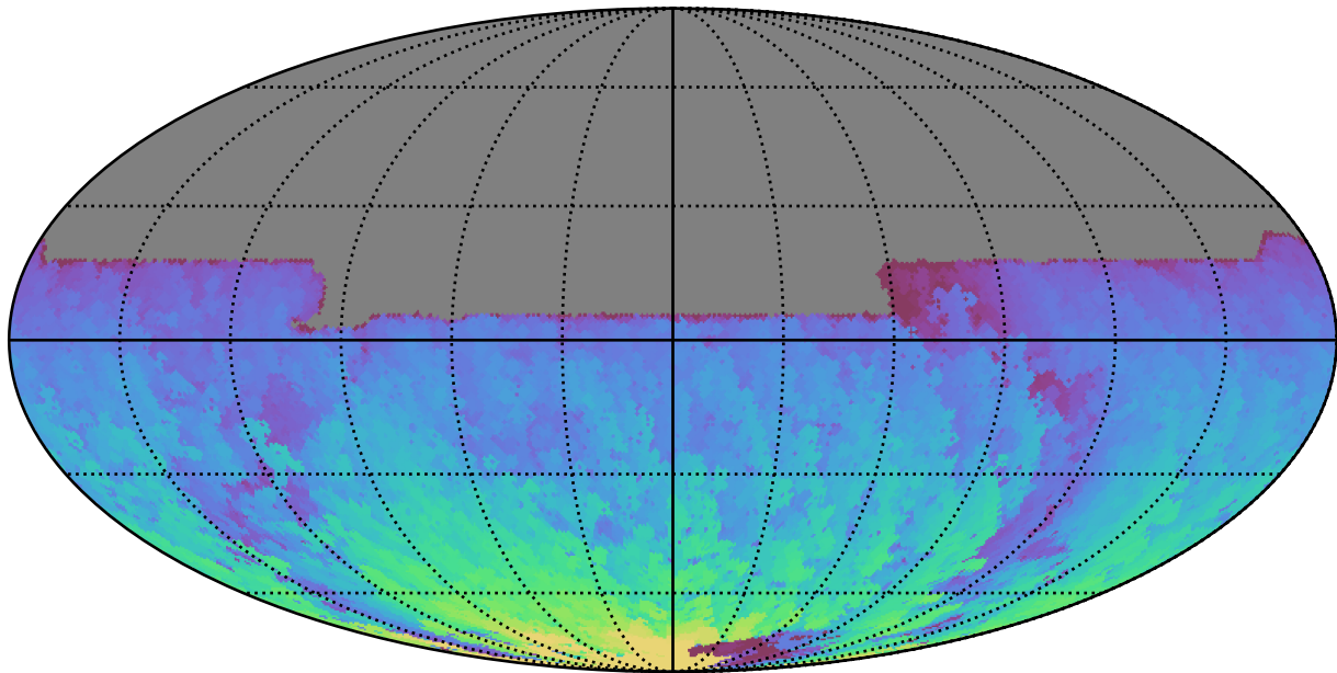
baseline_v3.5_10yrs All sky y band: Max HA
