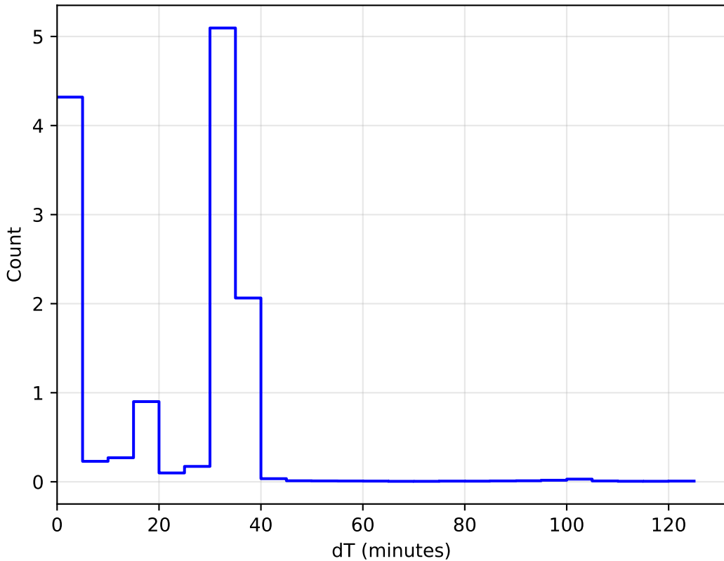
1e6 baseline_v3.5_10yrs All sky: DeltaT Histogram
