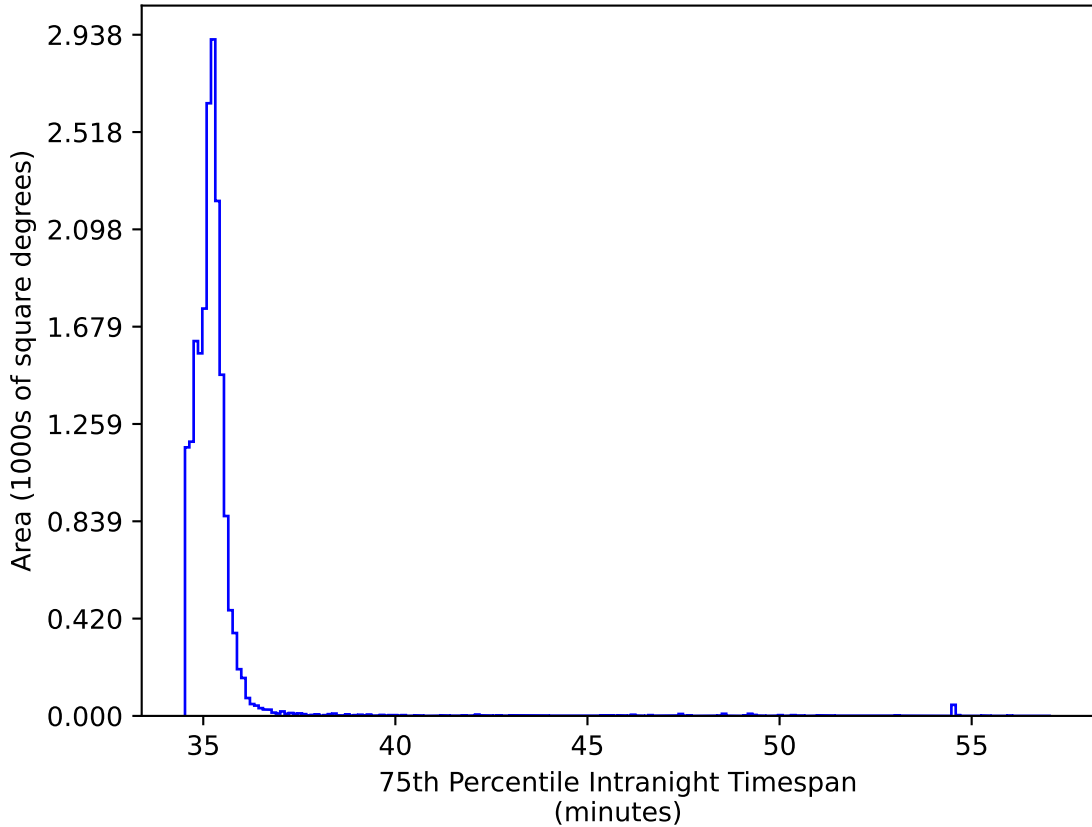
baseline_v3.5_10yrs WFD iz bands: 75th Percentile Intranight Timespan
