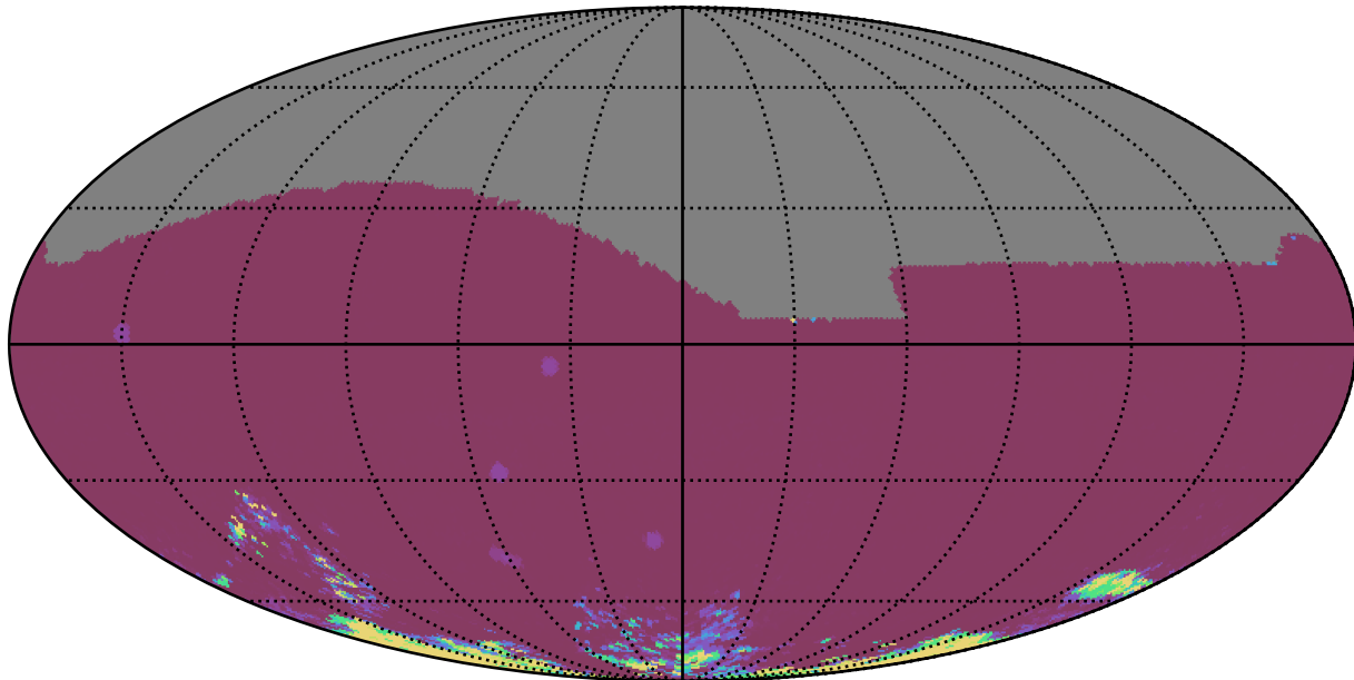
baseline_v3.5_10yrs All sky iz bands: 75th Percentile Intranight Timespan
