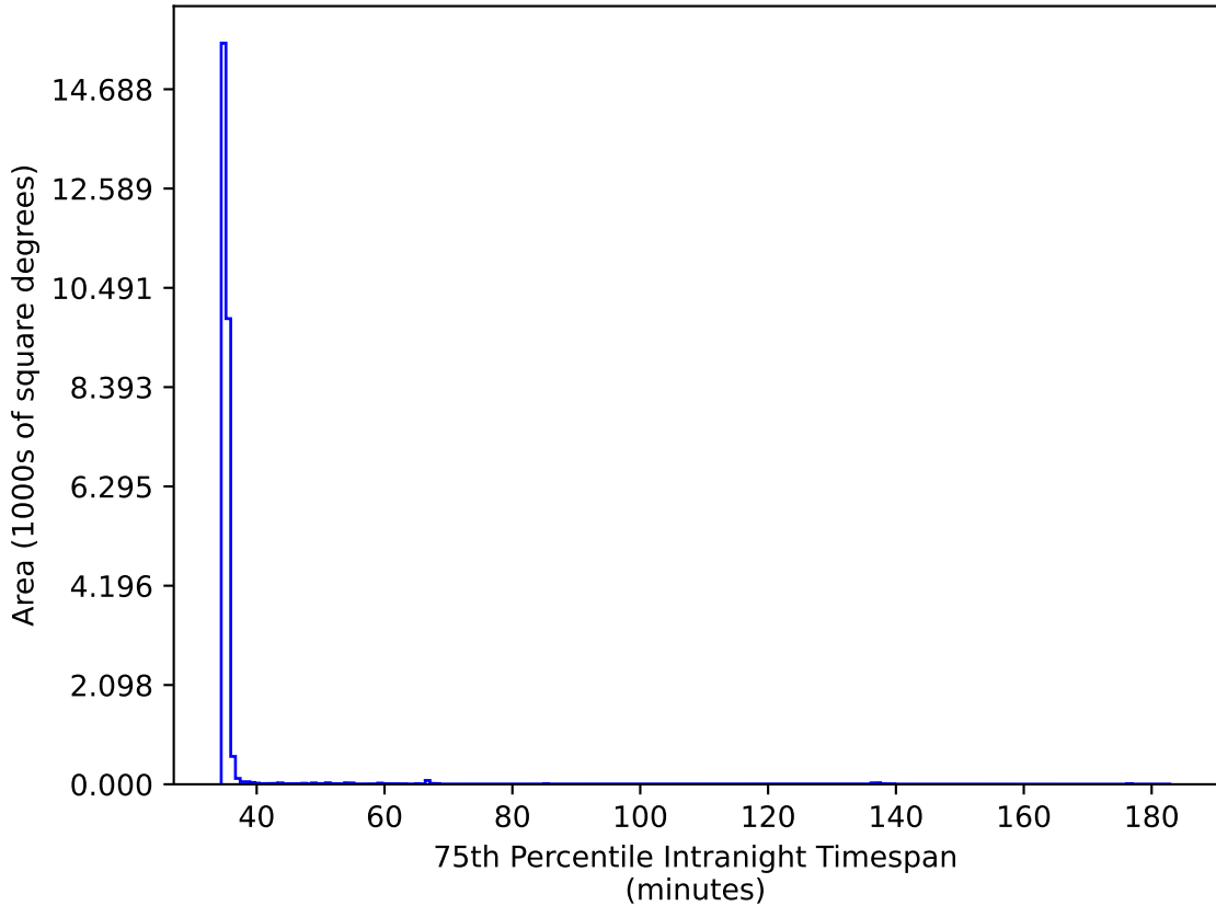
baseline_v3.5_10yrs All sky iz bands: 75th Percentile Intranight Timespan
