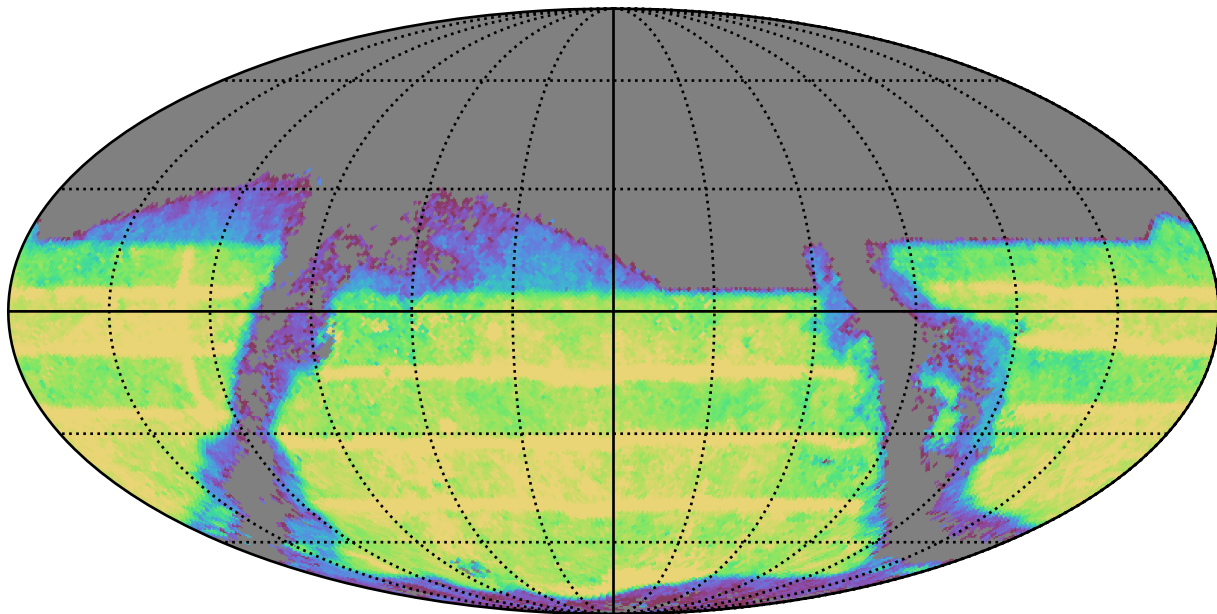
baseline_v3.4_10yrs : TDC_rate
