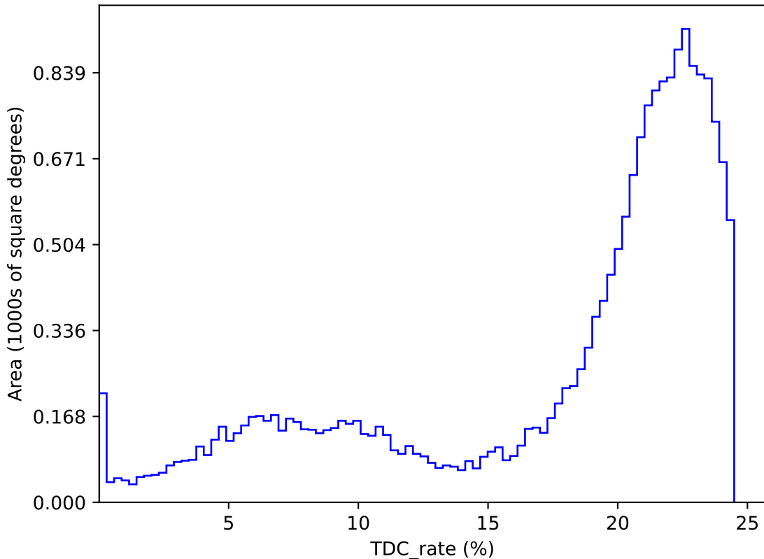
baseline_v3.4_10yrs : TDC_rate
