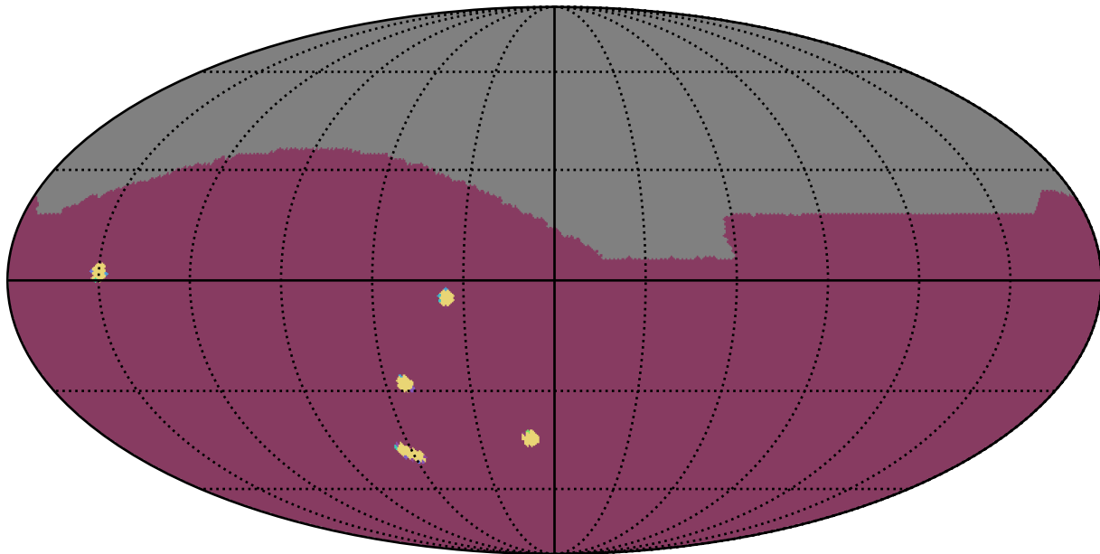
baseline_v3.4_10yrs : NumberOfQuickRevisits
