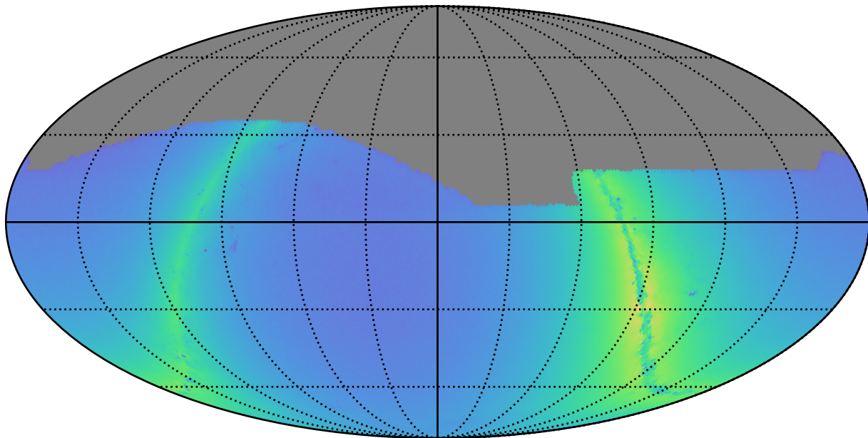
baseline_v3.4_10yrs i: Nstars_no_crowding
