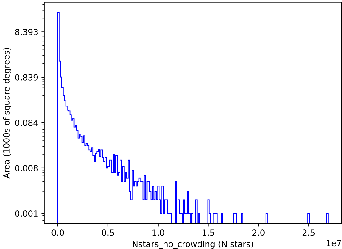
baseline_v3.4_10yrs i: Nstars_no_crowding
