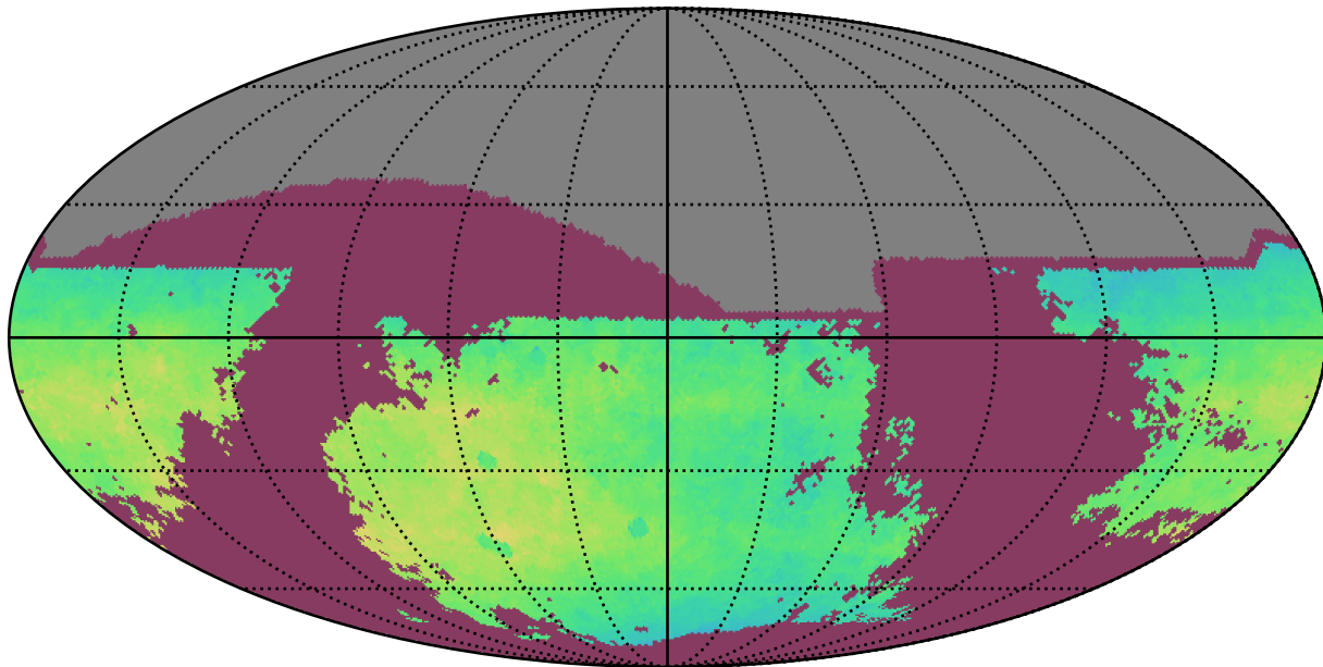
baseline_v3.4_10yrs i: NgalScale
