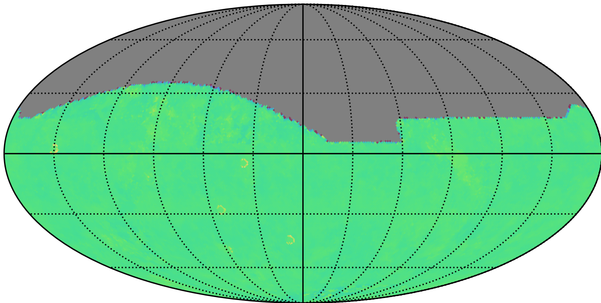
baseline_v3.4_10yrs z: Kuiper rotTelPos
