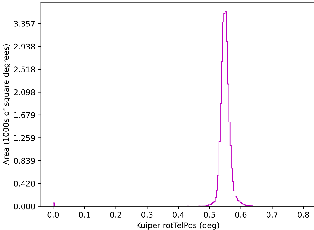
baseline_v3.4_10yrs z: Kuiper rotTelPos
