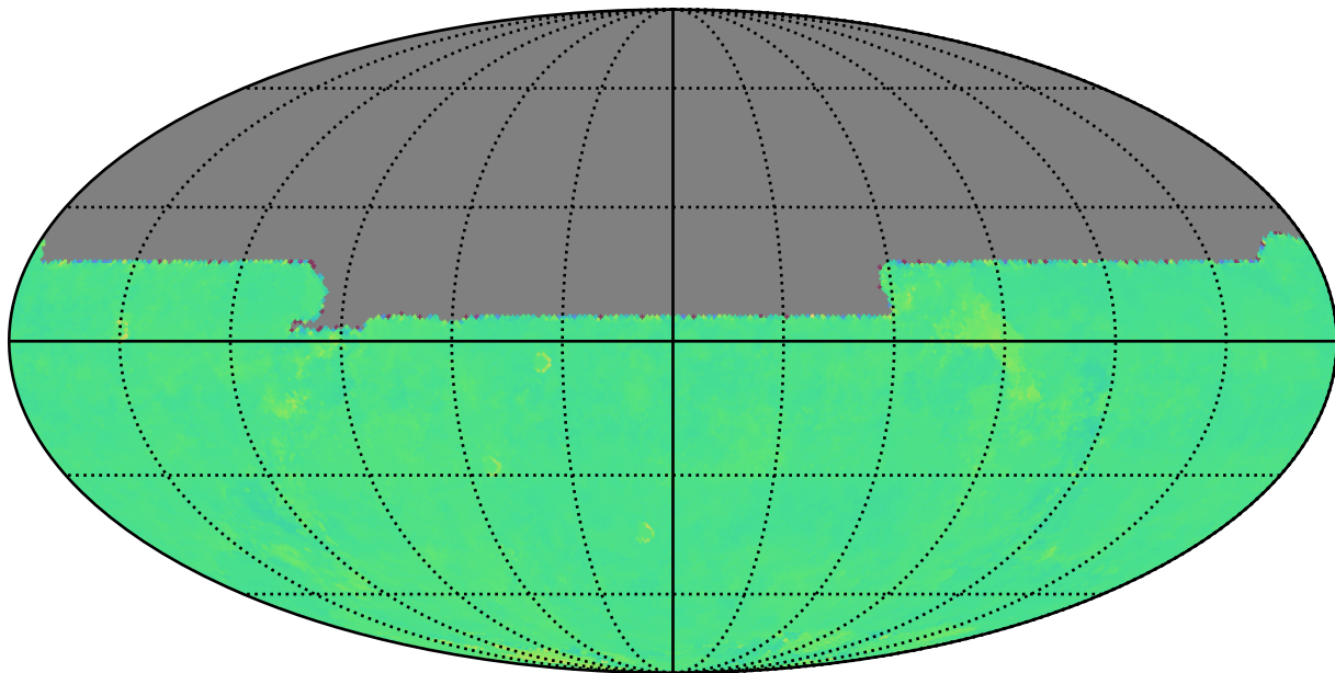
baseline_v3.4_10yrs y: Kuiper rotTelPos
