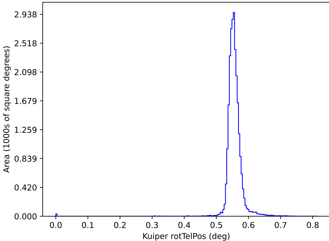
baseline_v3.4_10yrs y: Kuiper rotTelPos
