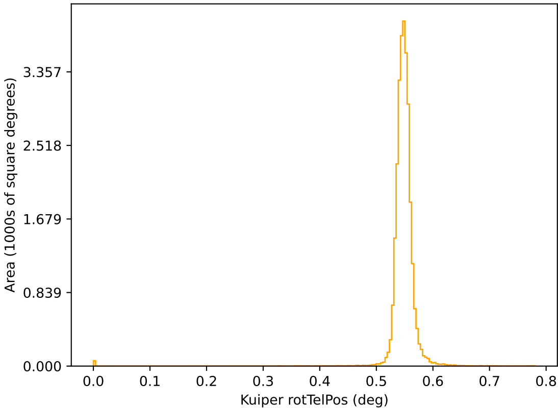
baseline_v3.4_10yrs r: Kuiper rotTelPos
