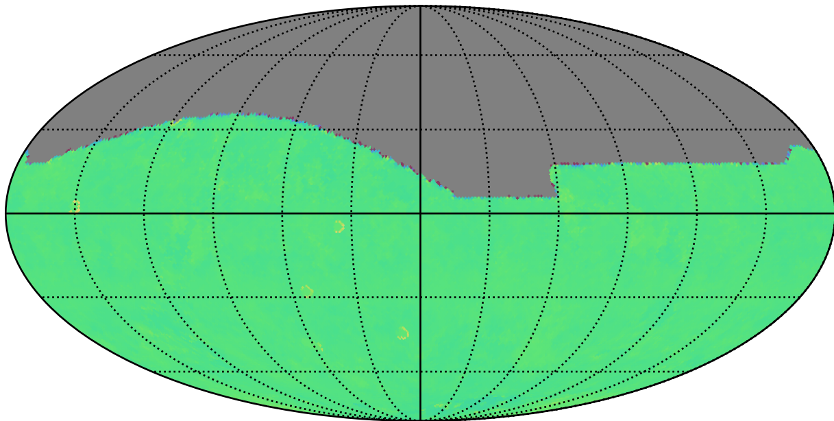
baseline_v3.4_10yrs i: Kuiper rotTelPos
