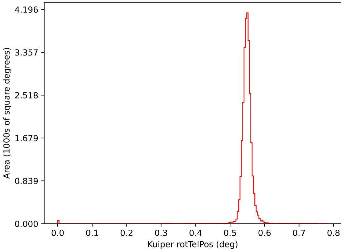
baseline_v3.4_10yrs i: Kuiper rotTelPos
