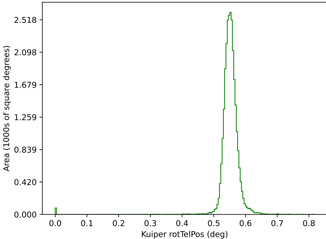
baseline_v3.4_10yrs g: Kuiper rotTelPos
