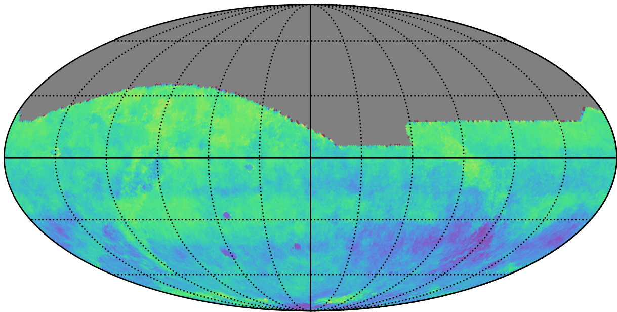
baseline_v3.4_10yrs z: Kuiper rotSkyPos
