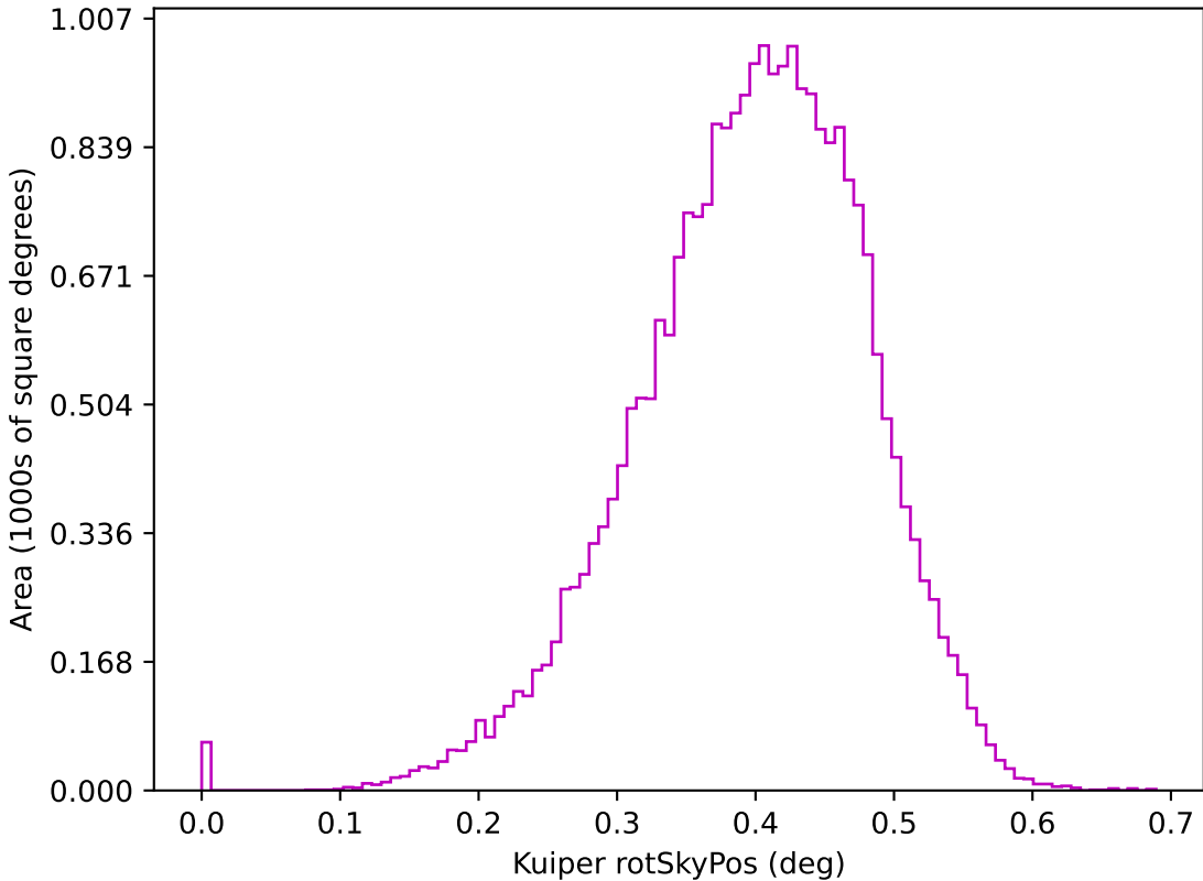
baseline_v3.4_10yrs z: Kuiper rotSkyPos
