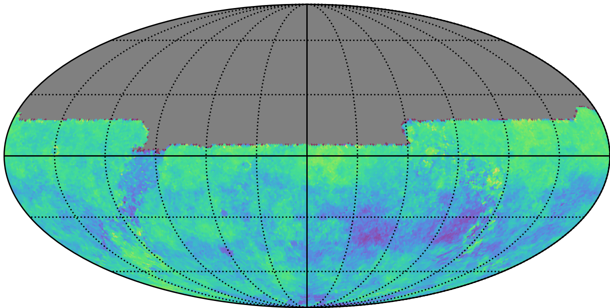
baseline_v3.4_10yrs u: Kuiper rotSkyPos
