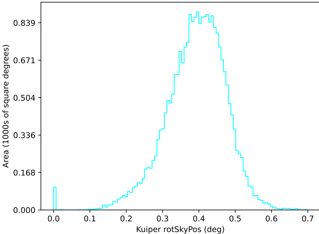
baseline_v3.4_10yrs u: Kuiper rotSkyPos
