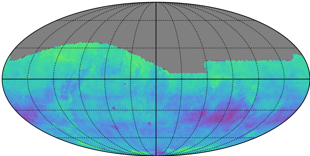
baseline_v3.4_10yrs r: Kuiper rotSkyPos
