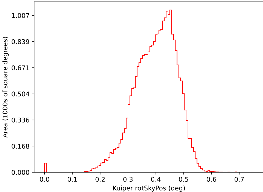
baseline_v3.4_10yrs i: Kuiper rotSkyPos
