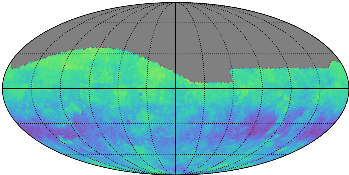
baseline_v3.4_10yrs g: Kuiper rotSkyPos
