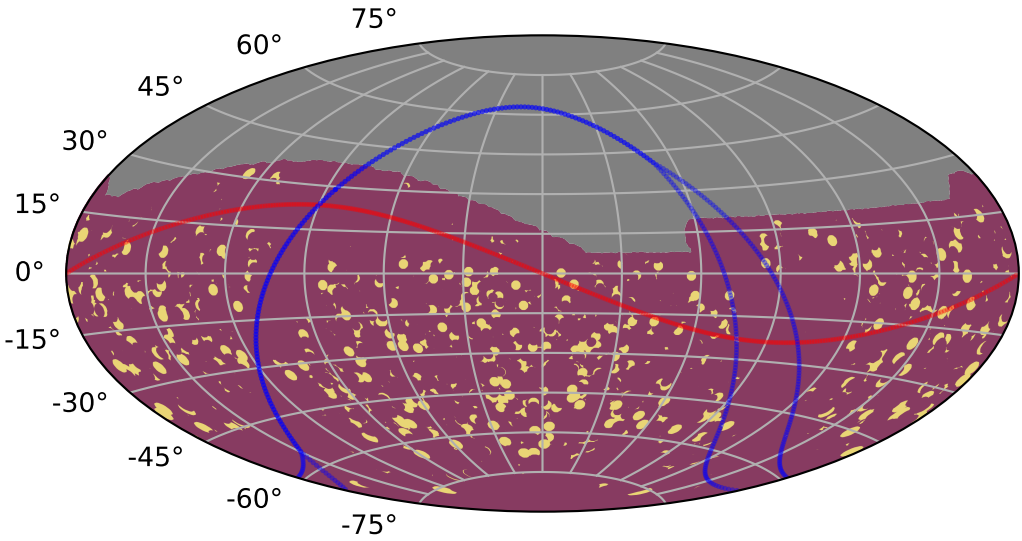
baseline_v3.4_10yrs all models: KNePopMetric_all_multi_detect
