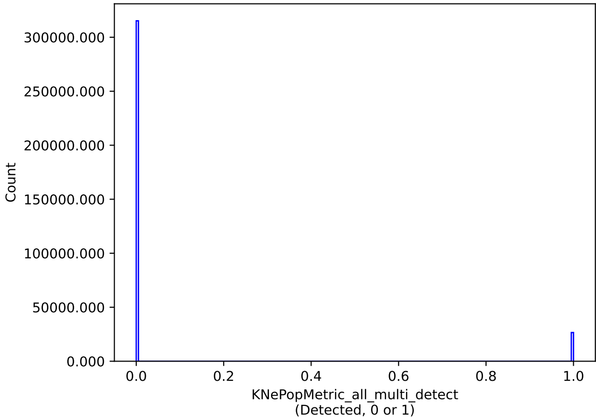
baseline_v3.4_10yrs all models: KNePopMetric_all_multi_detect
