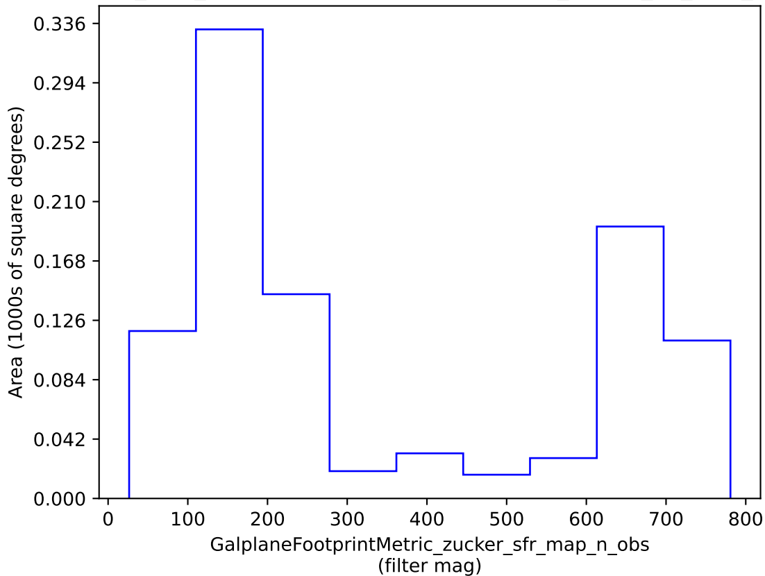
baseline_v3.4_10yrs : GalplaneFootprintMetric_zucker_sfr_map_n_obs
