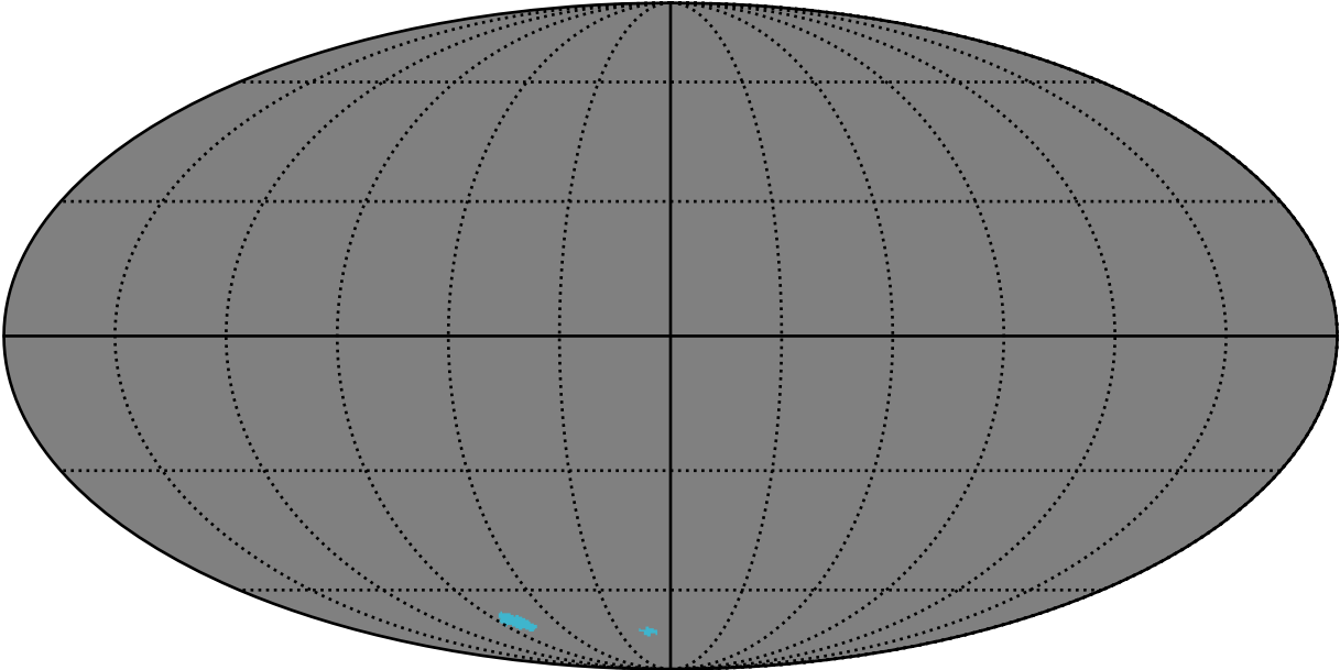
baseline_v3.4_10yrs : GalplaneFootprintMetric_magellanic_clouds_map_Tau_5_0
