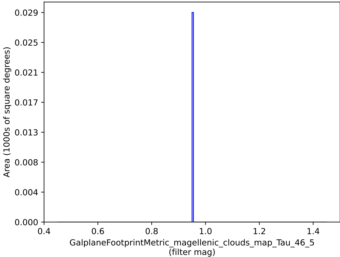
baseline_v3.4_10yrs : GalplaneFootprintMetric_magellanic_clouds_map_Tau_46_5
