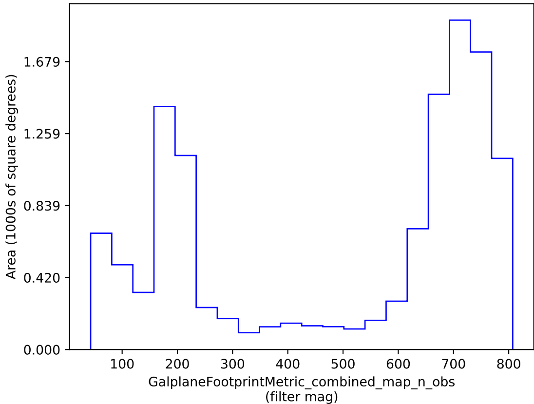
baseline_v3.4_10yrs : GalplaneFootprintMetric_combined_map_n_obs
